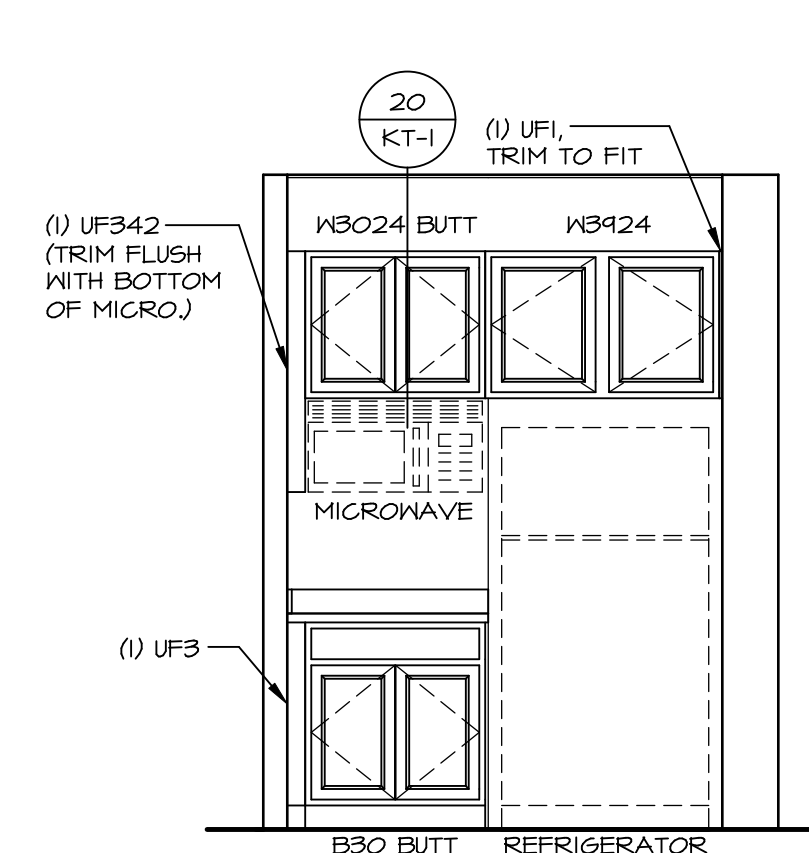
E CABINET ELEVATION SCALE: 3/8" = 1'-0"
