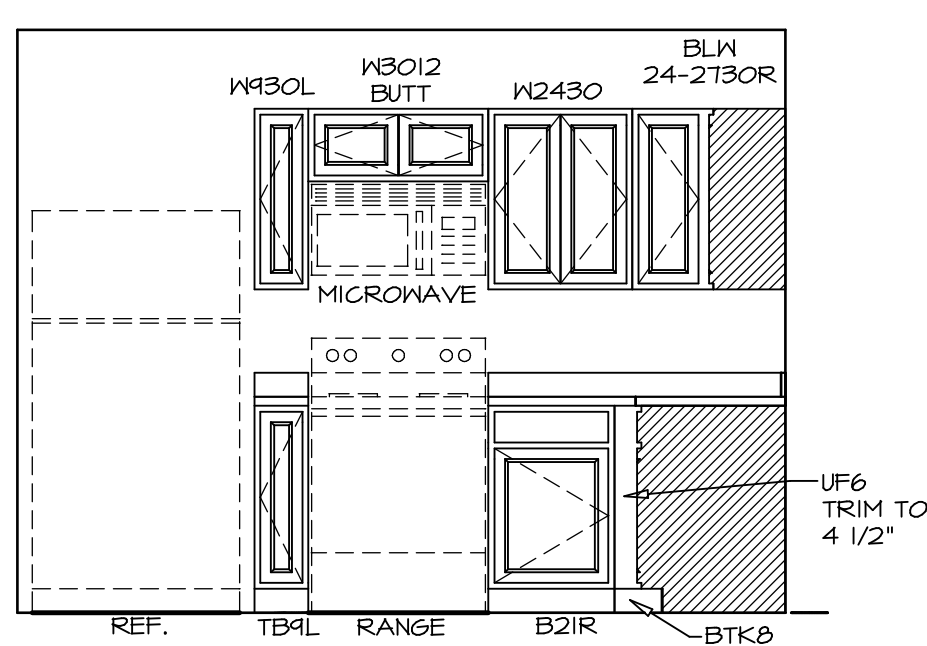
A ELEVATION SCALE: 3/8" = 1'-0"
