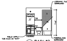
F BATH #2 SCALE: 1/4" = 1'-0"
