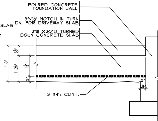
SCALE: 1/4" = 1'-0"
