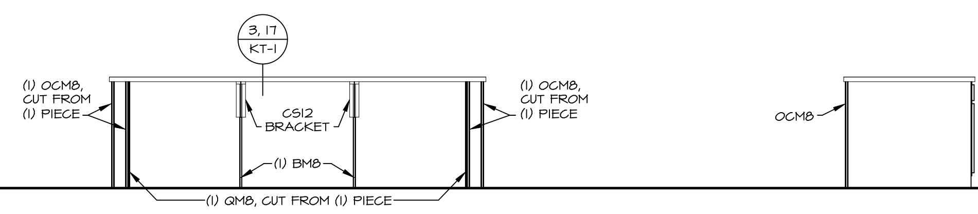
D CABINET ELEVATION SCALE: 3/8" = 1'-0"
