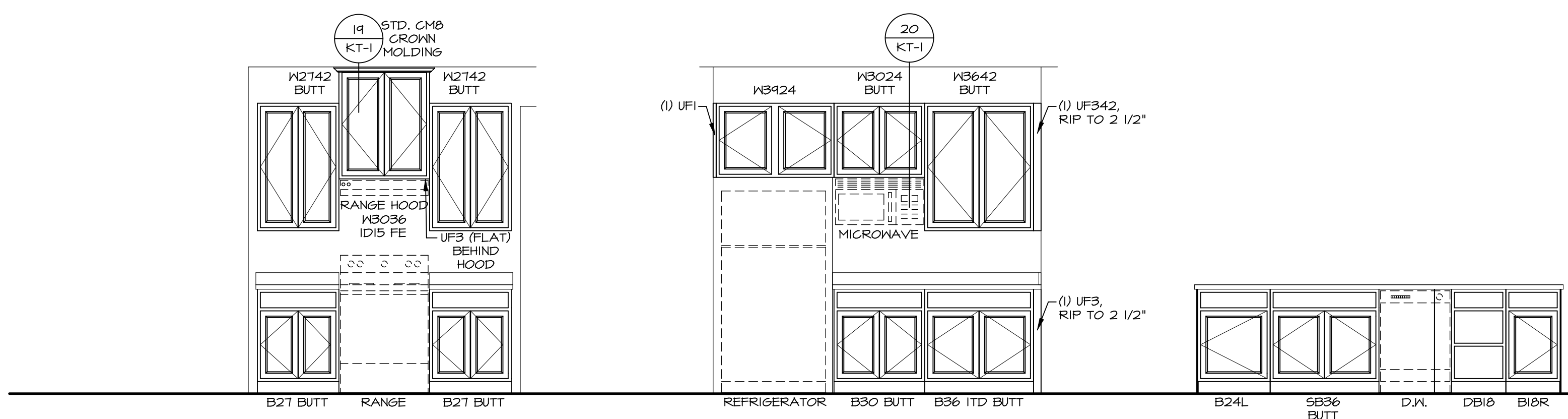
A CABINET ELEVATION SCALE: 3/8" = 1'-0"
