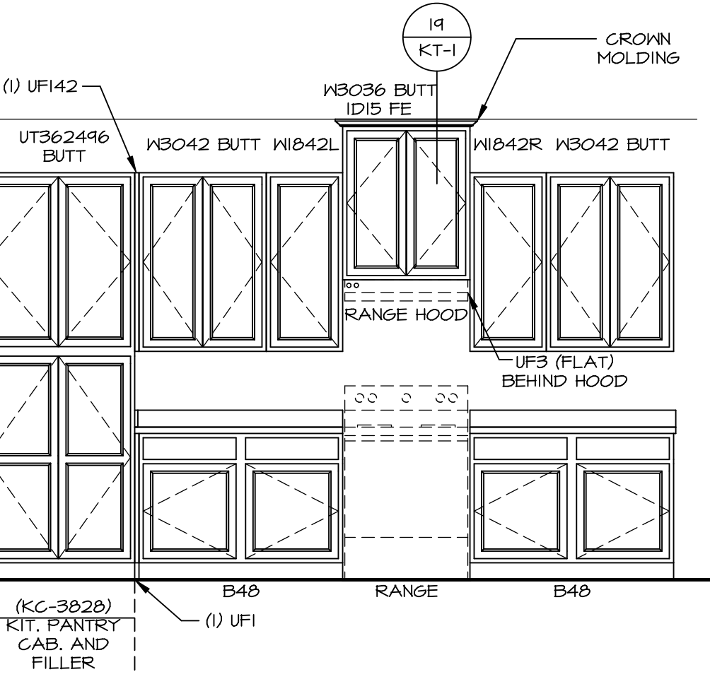
A CABINET ELEVATION SCALE: 3/8" = 1'-0"
